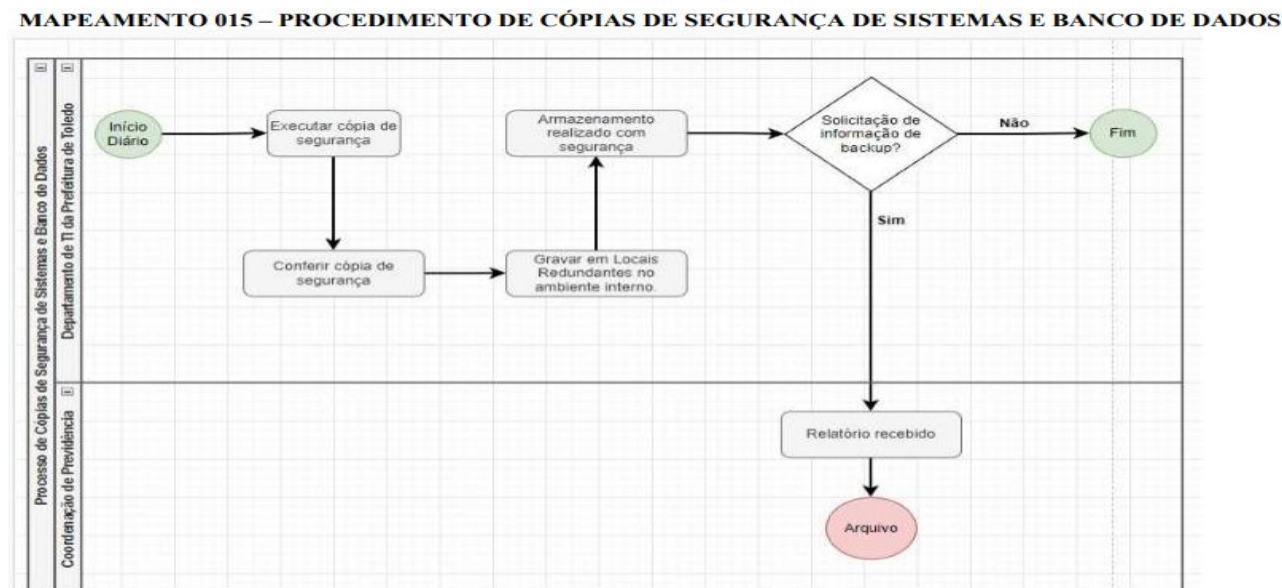
Figura 15 – Procedimentos de Cópias de Segurança de Sistemas e Banco de Dados 34 .
