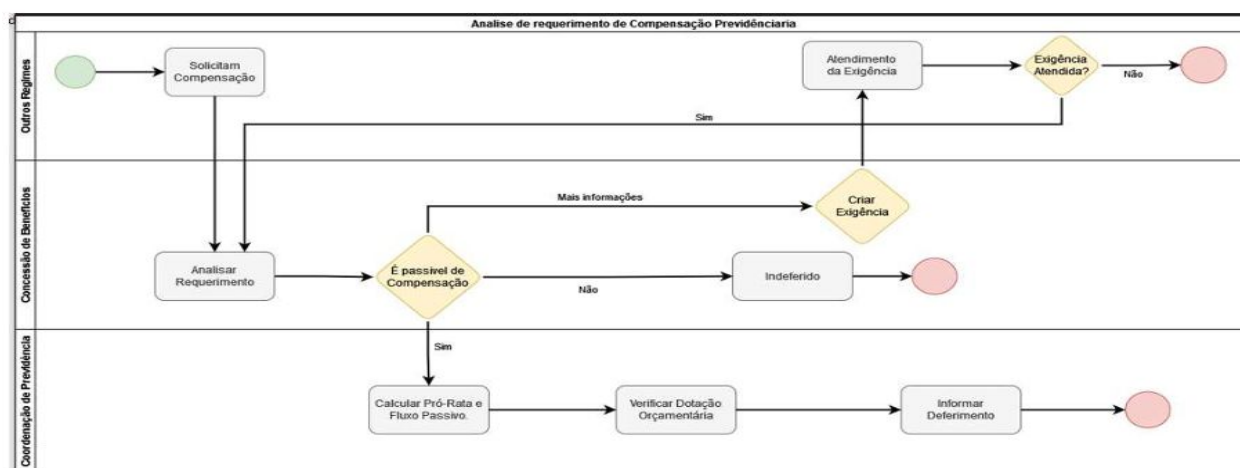
Figura 16 – Análise de Requerimento de Compensação Previdenciária 25
