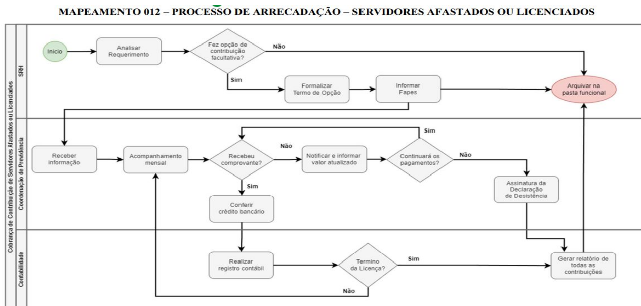
Figura 12 – Mapeamento do processo de arrecadação – Servidor Afastado ou Licenciado 19 .
