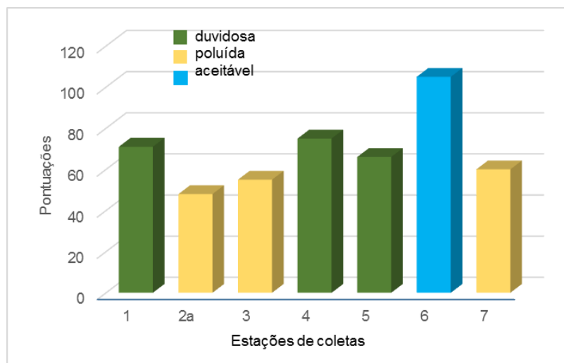
Figura 2.01 – Perfil da Qualidade Hídrica das Estações de Coleta de Macroinvertebrados Aquáticos em Toledo
