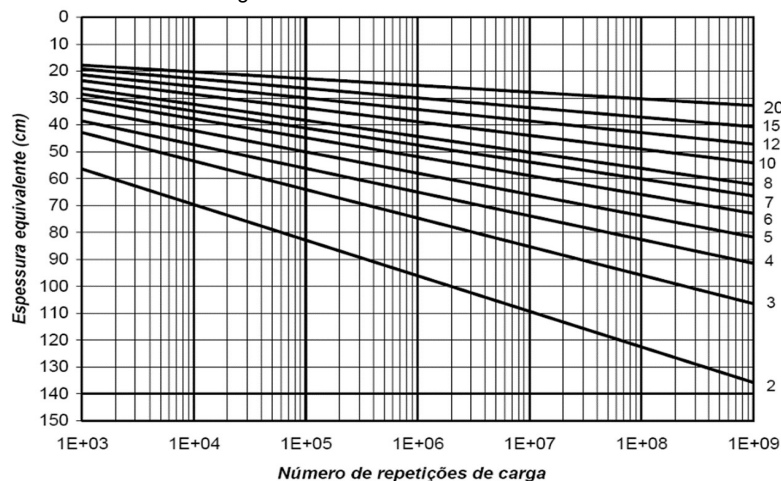
Figura 1 - Ábaco de dimensionamento
