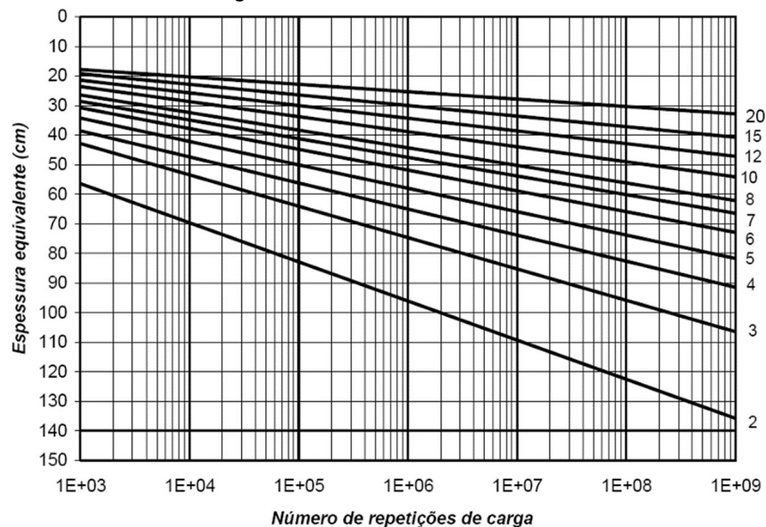
Figura 2 - Ábaco de dimensionamento
